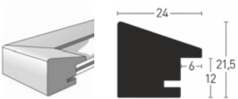
Max. Einlegehöhe 2,6 mm | Max. insertion height 2,6 mm
